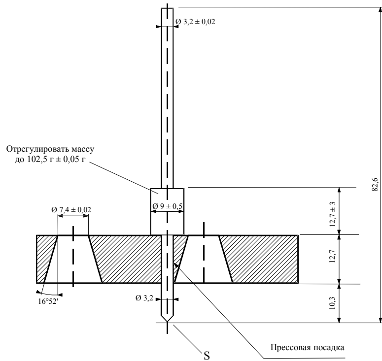
Рис. 1. Пенетрометр
