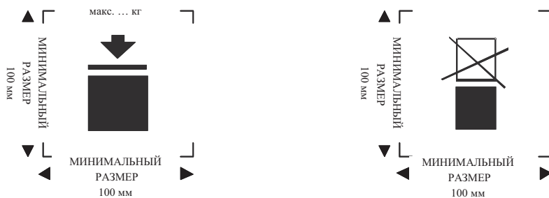
КСГМГ, выдерживающие штабелирование
