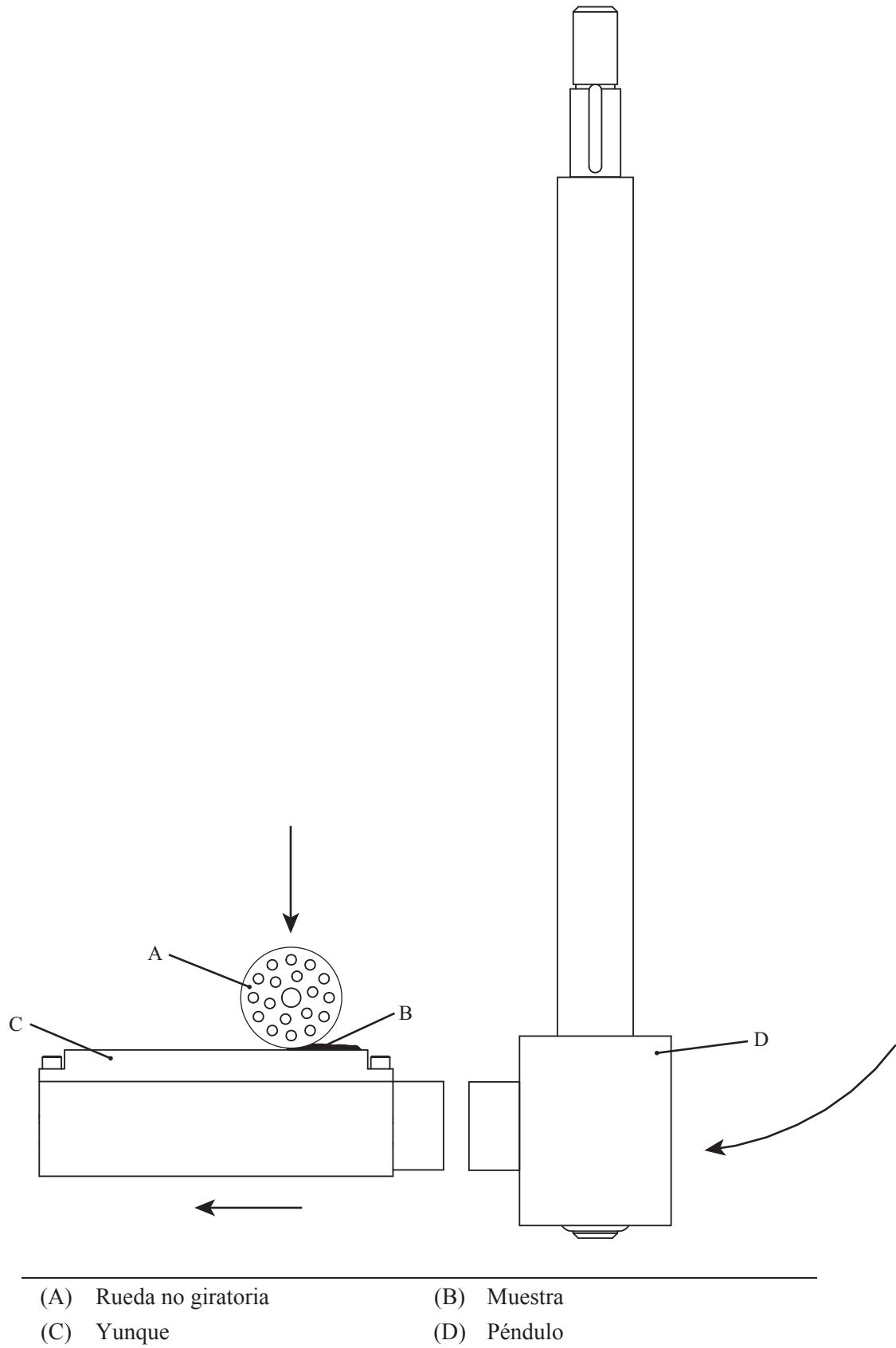
Figura 13.5.4.1: MÁQUINA DE FRICCIÓN ABL
