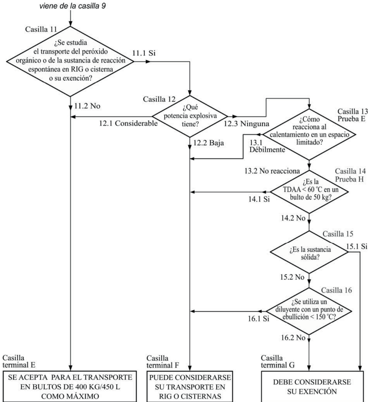
Figura 20.1 (b): DIAGRAMA-CUESTIONARIO PARA LAS SUSTANCIAS DE REACCIÓN ESPONTÁNEA Y LOS PERÓXIDOS ORGÁNICOS (continuación)
