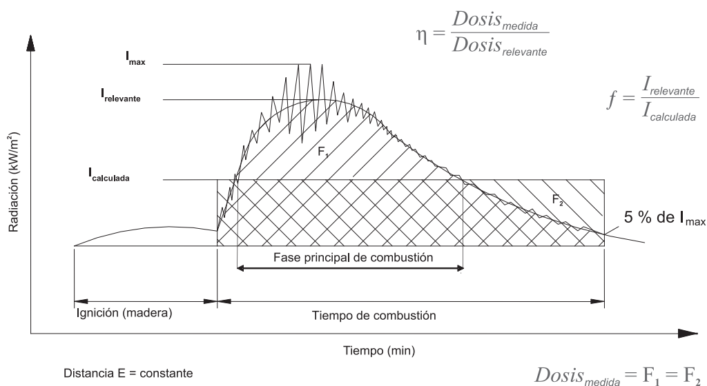
Figura 51.4.1: Medición de radiación en función del tiempo
