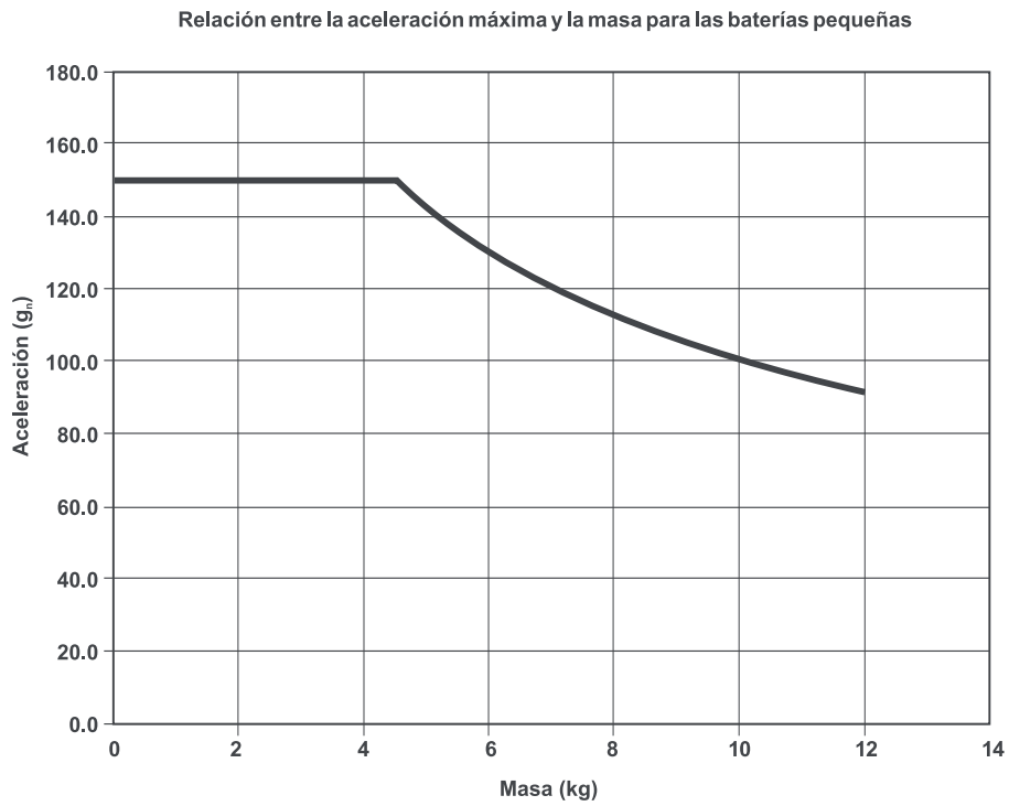
Figura 38.3.4.1: RELACIÓN ENTRE LA ACELERACIÓN MÁXIMA Y LA MASA PARA LAS BATERÍAS PEQUEÑAS (MENOS DE 12,0 Kg)
