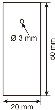
Figura 37.4.2.1: PROBETA
