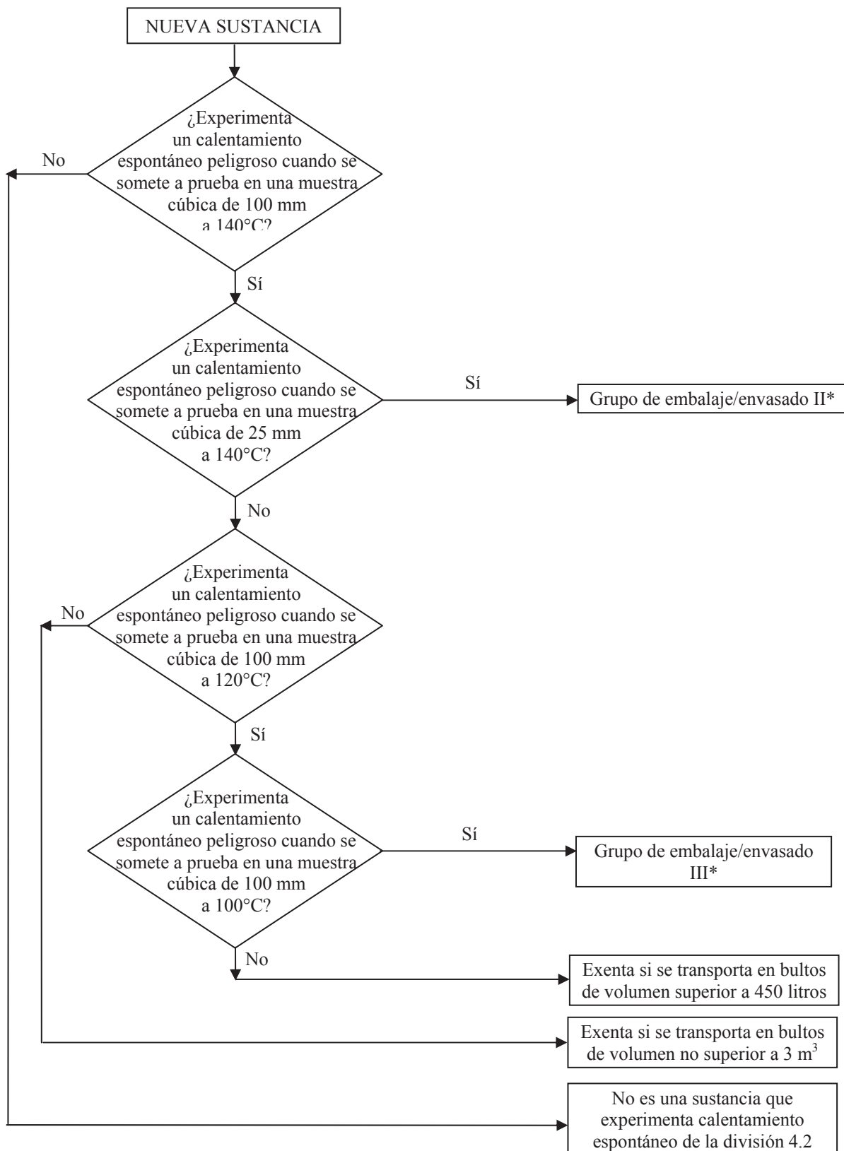
Figura 33.3.1.3.3.1: CLASIFICACIÓN DE LAS SUSTANCIAS QUE EXPERIMENTAN CALENTAMIENTO ESPONTÁNEO
