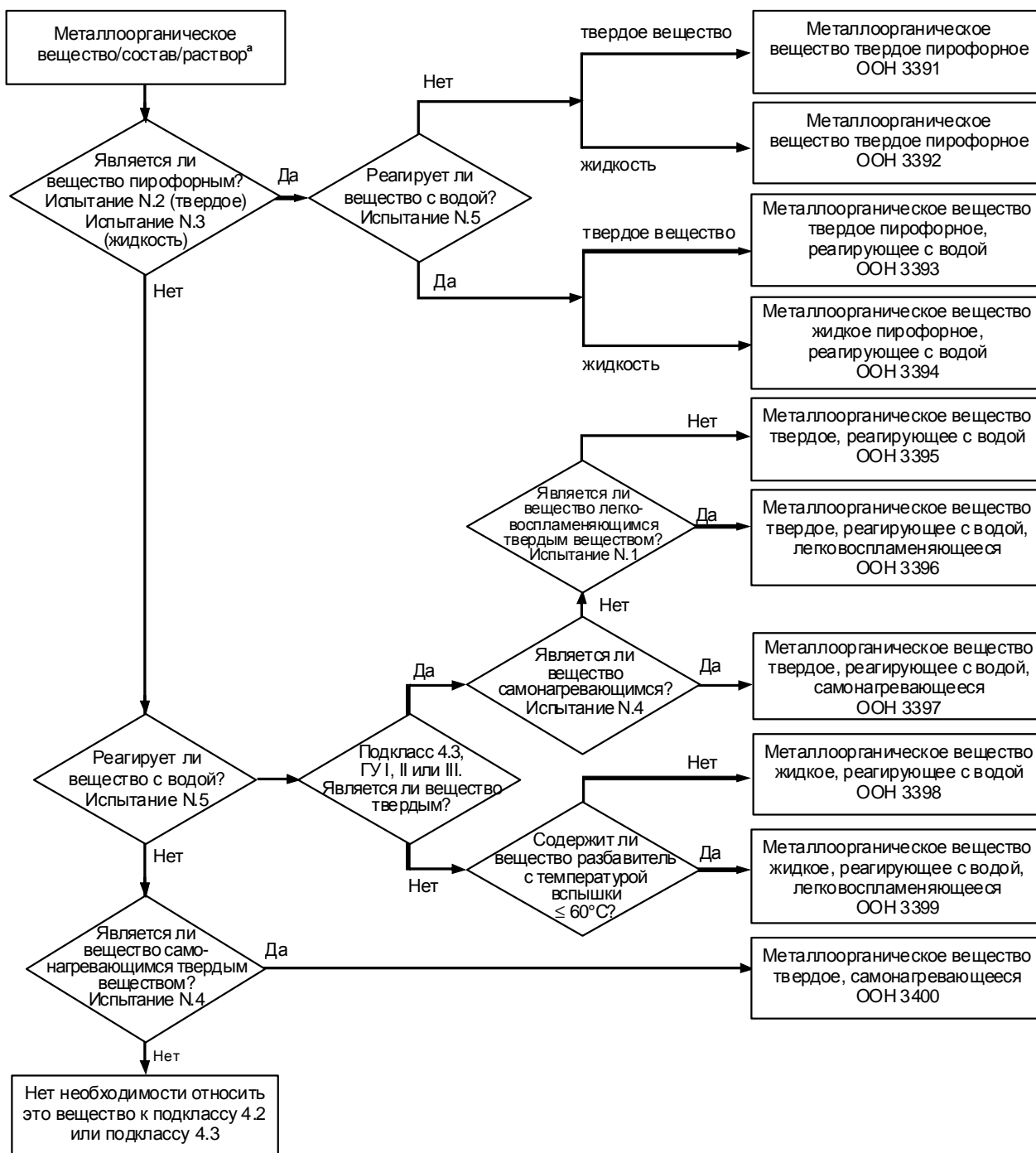
Рис. 2.4.2: СХЕМА КЛАССИФИКАЦИЯ МЕТАЛЛООРГАНИЧЕСКИХ ВЕЩЕСТВ b
