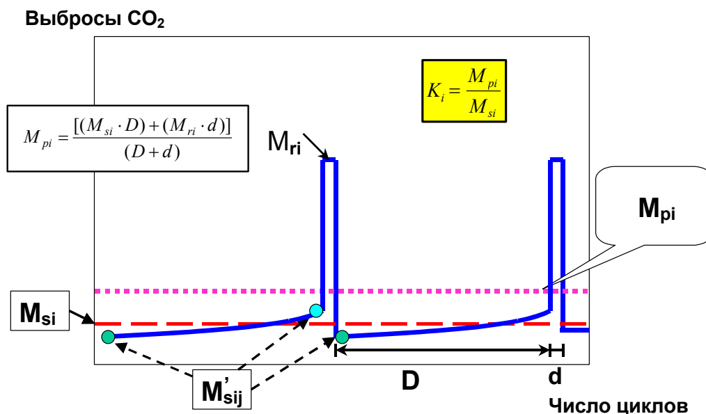
Рисунок 10/1 : Параметры, измеряемые в ходе испытания на выбросы двуокиси углерода и расхода топлива в процессе осуществления циклов, в рамках которых происходит регенерация, и между этими циклами (примерная схема, уровень выбросов в процессе "D" может возрасть или уменьшаться)
