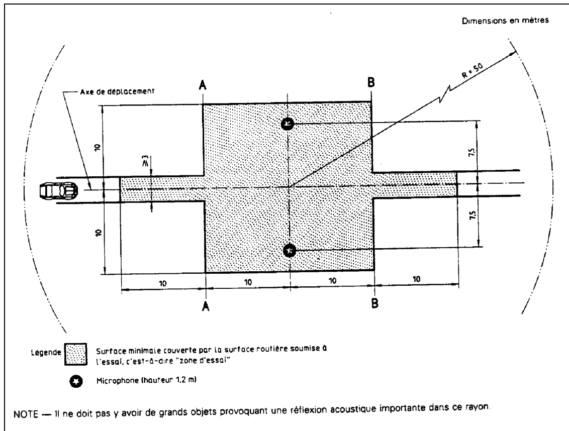
Figure 1 Prescriptions minimales concernant l'«aire d'essai» (zone ombrée)
