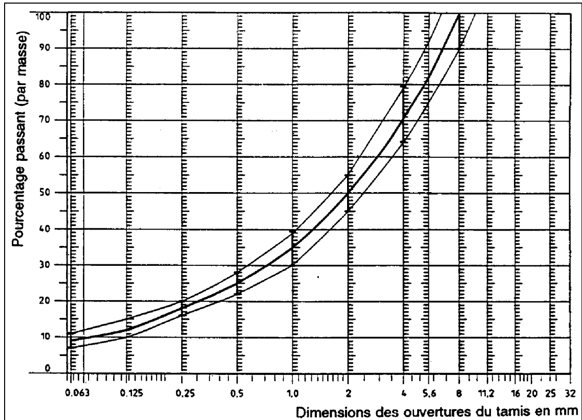
Figure 2 Courbe granulométrique des granulats enrobés, avec tolérances
