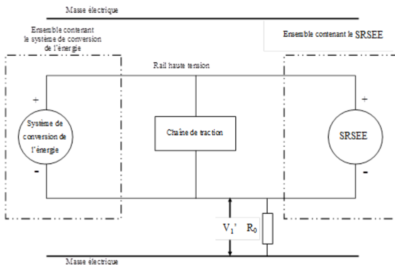
Figure 3 Mesure de V_1'
