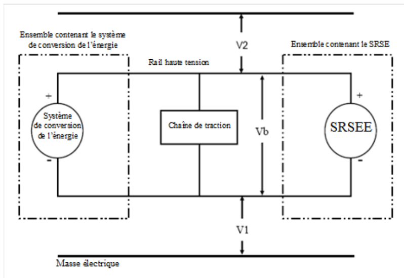
Figure 1 Mesure de V_b , V_1 et V_2
