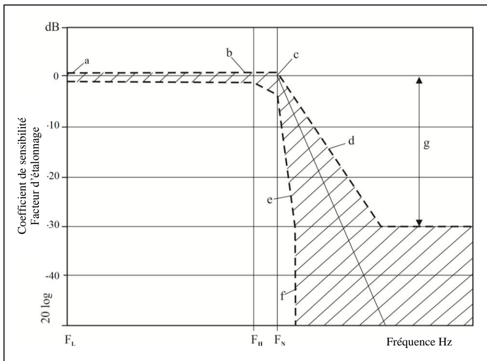
Figure 1 Courbe de réponse en fréquence
