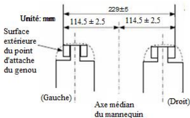
Figure 2 Distance initiale du genou pour le mannequin du type Hybrid III femme du cinquième centile
