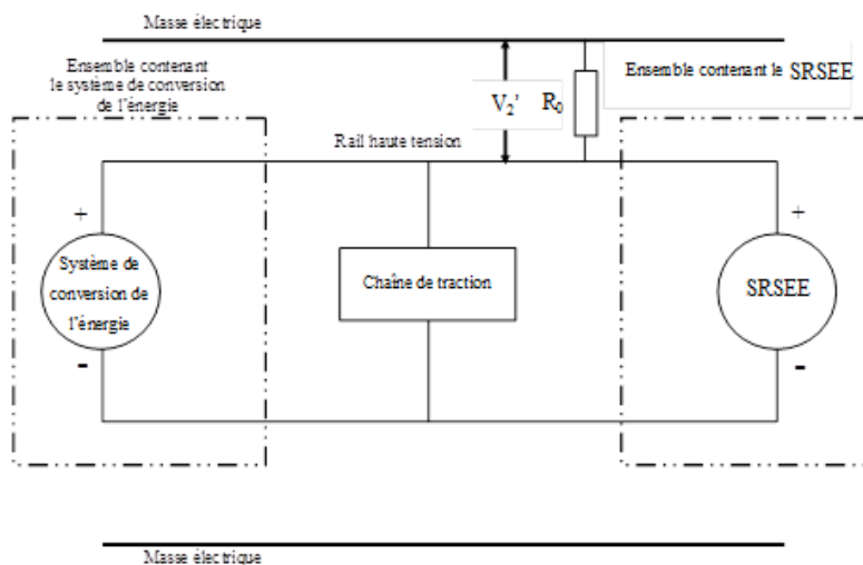
Figure 4 Mesure de V_2'
