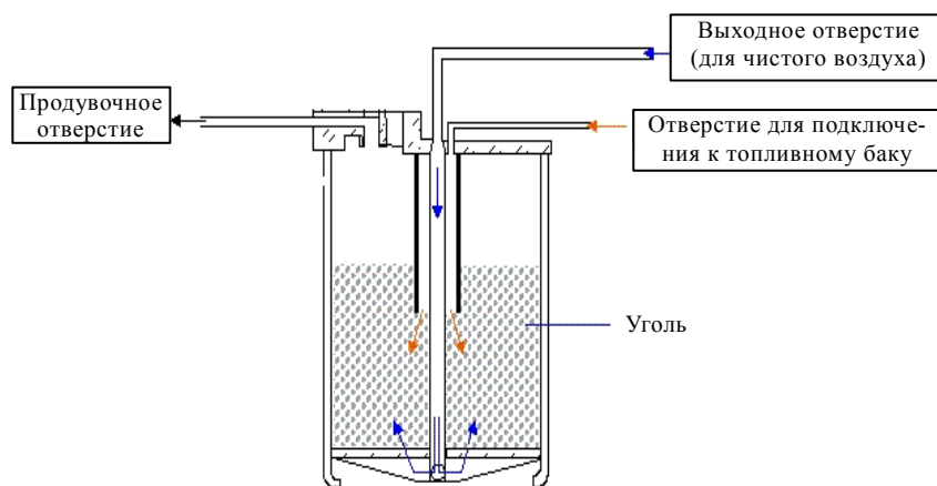
Схема газовых потоков и отверстия угольного фильтра
