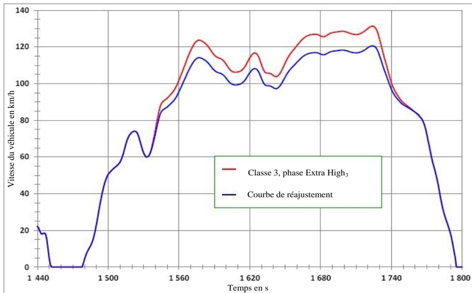
Figure A1/4516 Réajustement de la vitesse durant la phase à extra haute vitesse du cycle WLTC pour les véhicules de la classe 3
