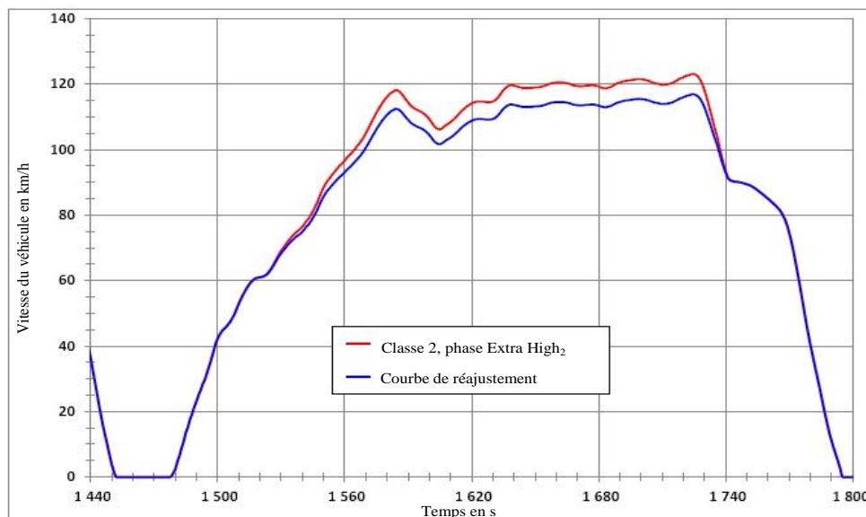
Figure A1/4415 Réajustement de la vitesse durant la phase à extra haute vitesse du cycle WLTC pour les véhicules de la classe 2
