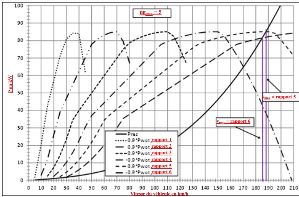
Figure 1b Cas où n_{g_{max}} est le rapport le plus élevé moins 1
