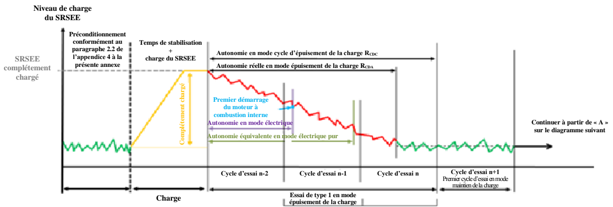
Temps de stabilisation entre cycles d'essai durant l'essai du type 1 en mode épuisement de la charge 30 min max.
