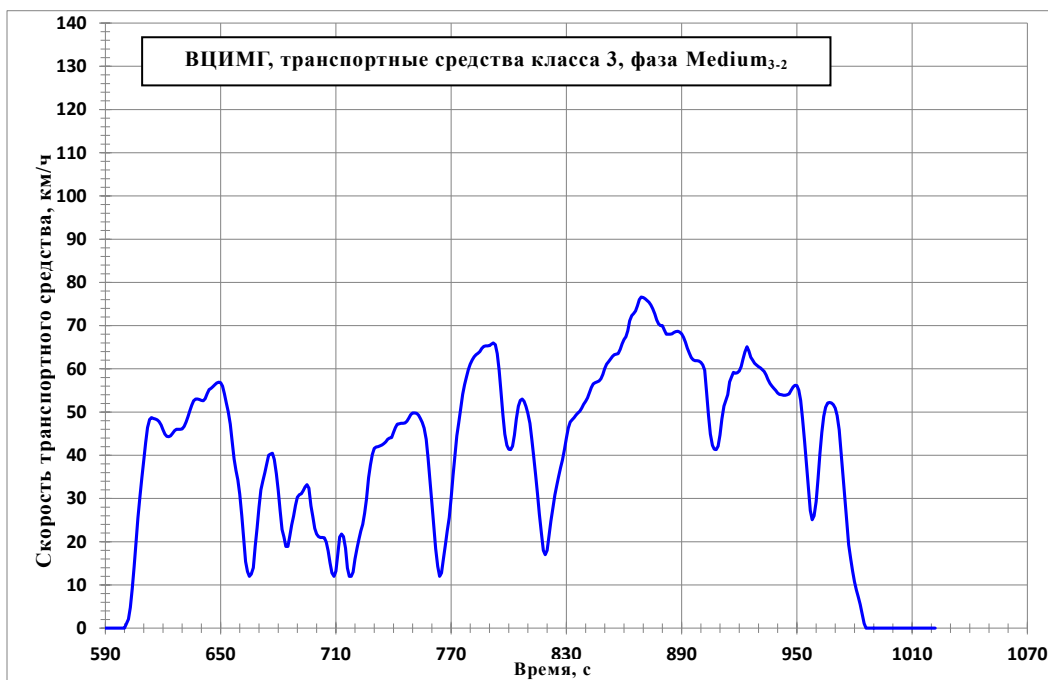
Рис. А1/9 ВЦИМГ, транспортные средства класса 3, фаза Medium 3-2
