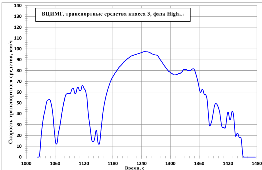
Рис. А1/10 ВЦИМГ, транспортные средства класса 3, фаза High 3-1
