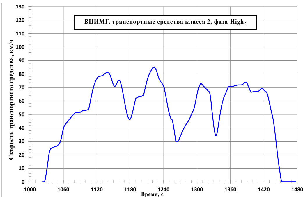
Рис. А1/5 ВЦИМГ, транспортные средства класса 2, фаза High 2
