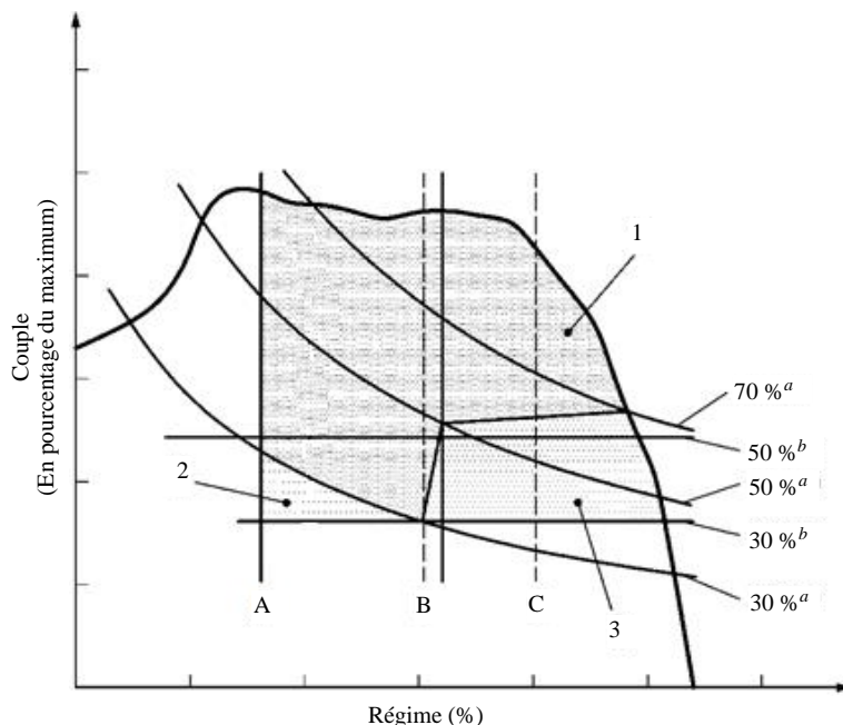
Figure 3 Plage de contrôle pour les moteurs à régime variable de la catégorie NRE ayant une puissance nette maximale inférieure à 19 kW et un régime C supérieur ou égal à 2 400 tr/min
