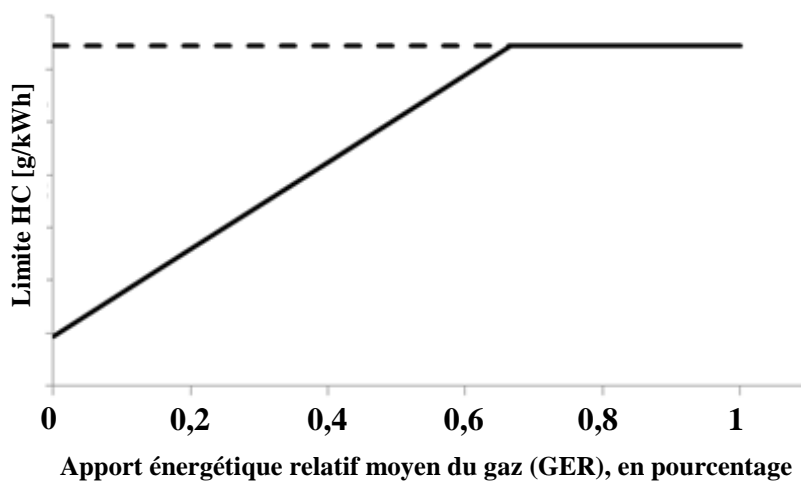
Figure 5 Diagramme montrant la limite des émissions de HC en fonction du GER moyen
