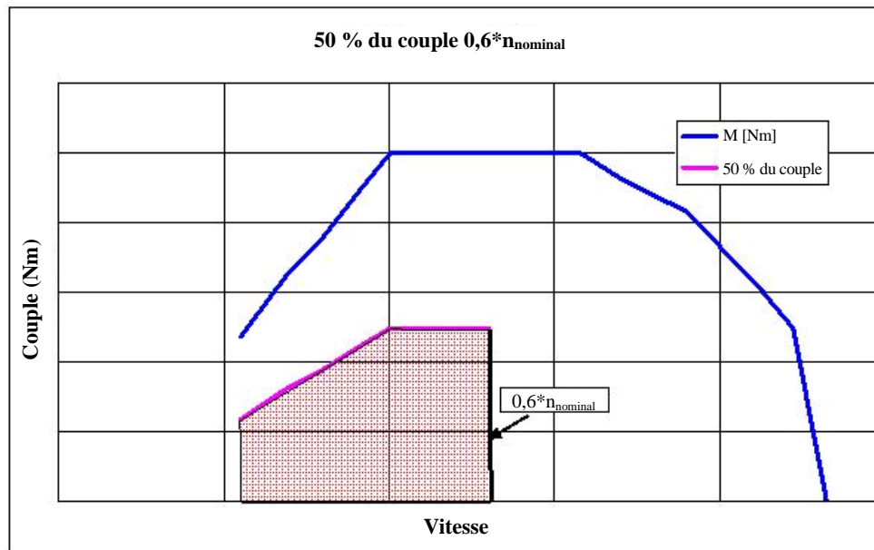
Figure A.9-2 Schéma de réduction du couple (incitation “sévère”)
