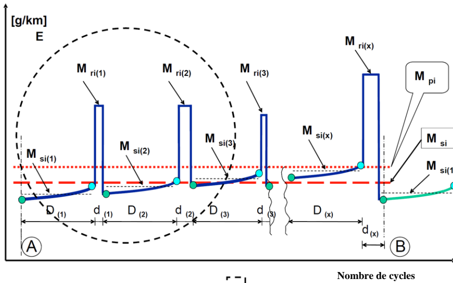
Figure A6.App1/2 Paramètres mesurés lors des essais d'émissions pendant et entre les cycles où se produit une régénération (il ne s'agit que d'un exemple)
