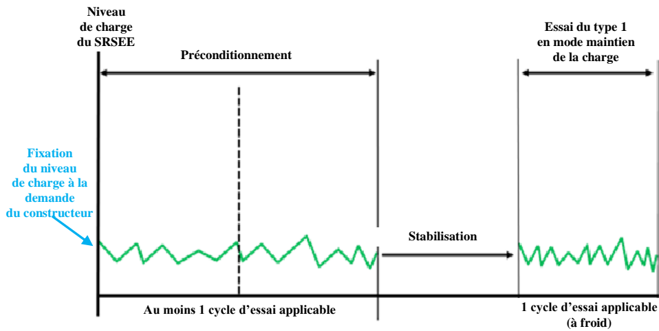
Figure A8.App1/2 VHE-RE, essai de maintien de la charge du type 1
