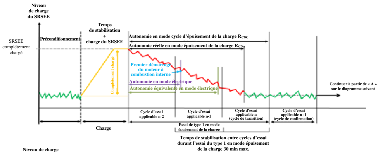
Figure A8.App1/3 VHE-RE, essai d'épuisement de la charge du type 1 suivi d'un essai de maintien de la charge du type 1
