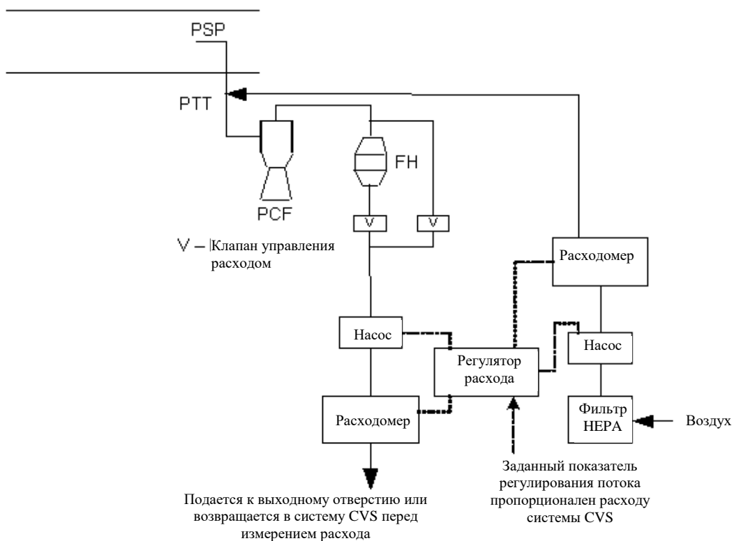
Рис. A5/13 Система отбора проб взвешенных частиц с двойным разбавлением
