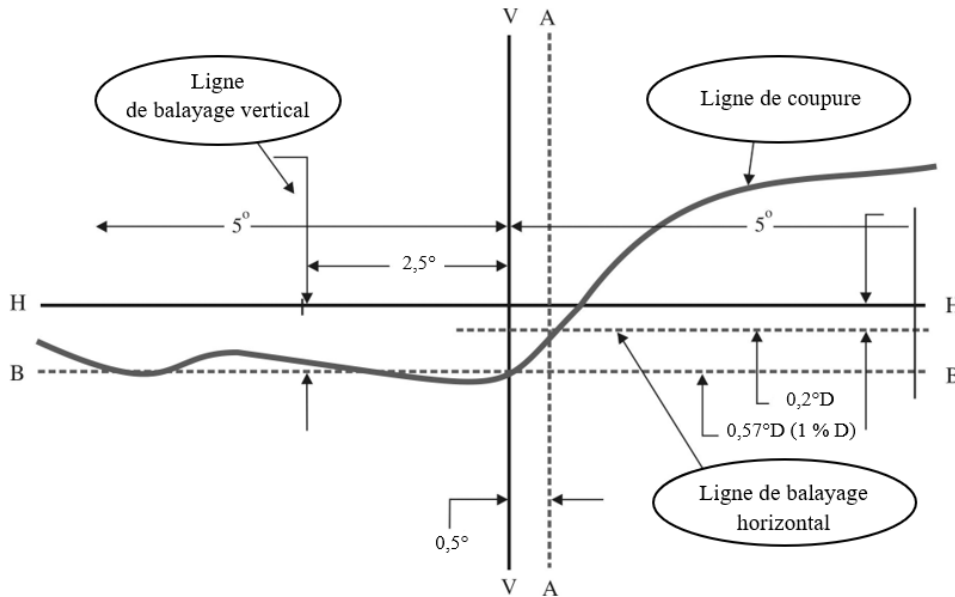
Figure A5-III Réglage instrumental vertical et horizontal – Méthode du balayage de la ligne horizontale
