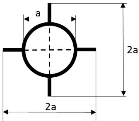
Figure A11-I Centre de référence
