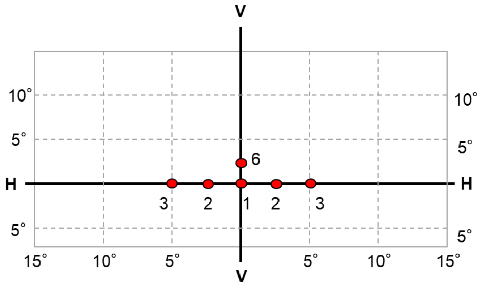
Figure A4-IV Position des points d'essai pour un faisceau de route secondaire
