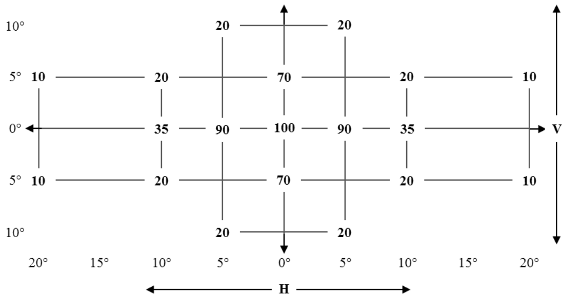
Figure A3-I Répartition normalisée de la lumière pour les feux de position avant et arrière, les feux de stationnement, les feux d'encombrement, les feux-stop et les feux indicateurs de direction
