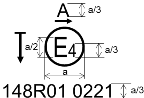
Figure A7-I – Exemple de marque 1
