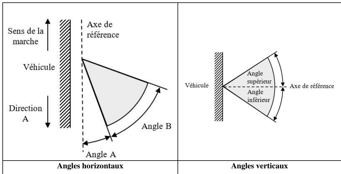
Figure A2-II Angles de visibilité géométrique horizontaux et verticaux
