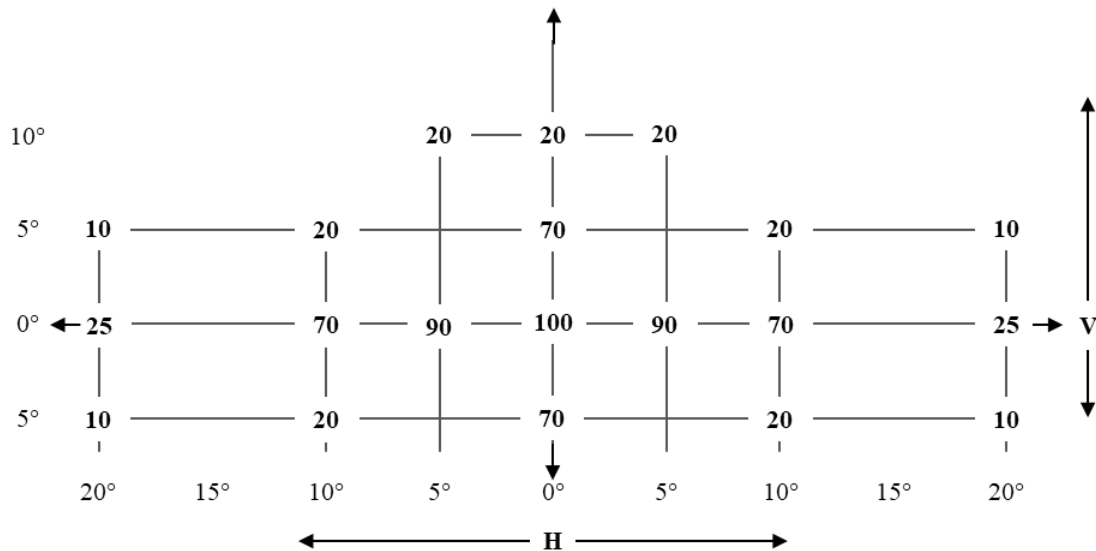
Figure A3-II Répartition de la lumière pour les feux de circulation diurne
