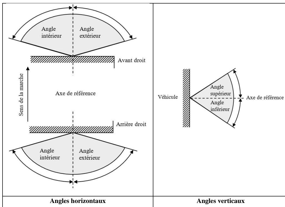
Figure A2-I Angles de visibilité géométrique horizontaux et verticaux
