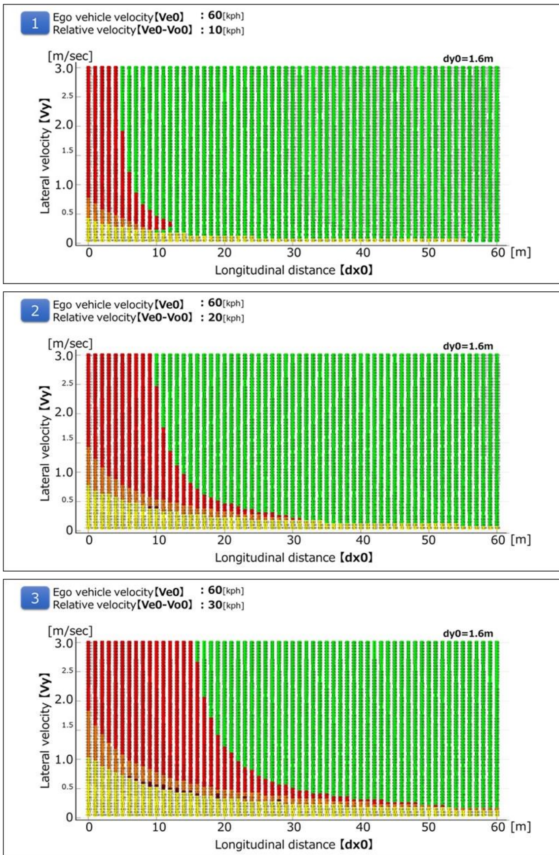
Рис. 8 Для V_{e0} = 60 км/ч
