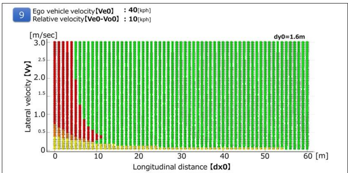
Рис. 10 Для V_{e0} = 40 км/ч
