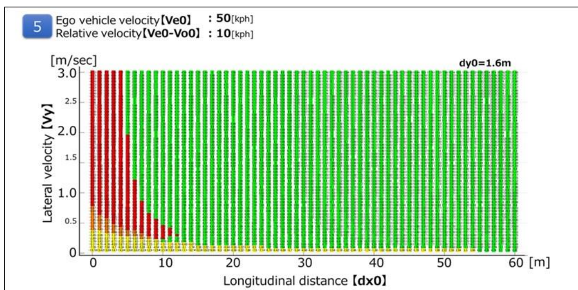
Рис. 9 Для V_{e0} = 50 км/ч
