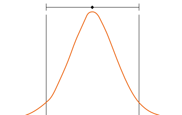
Рис. I – Понимание нормального (гауссова) распределения
