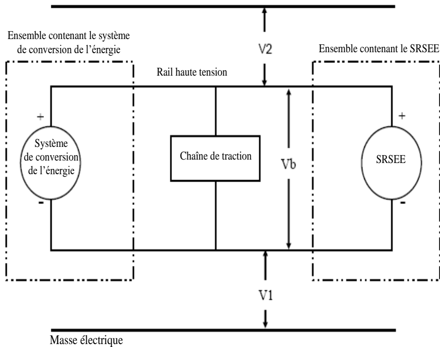
Figure 1 Mesure de V_b , V_1 et V_2
