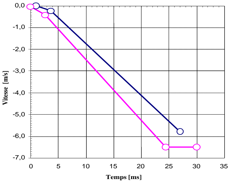
Figure 8 Rapport vitesse/temps du pendule pour l'essai d'homologation du rachis lombaire
