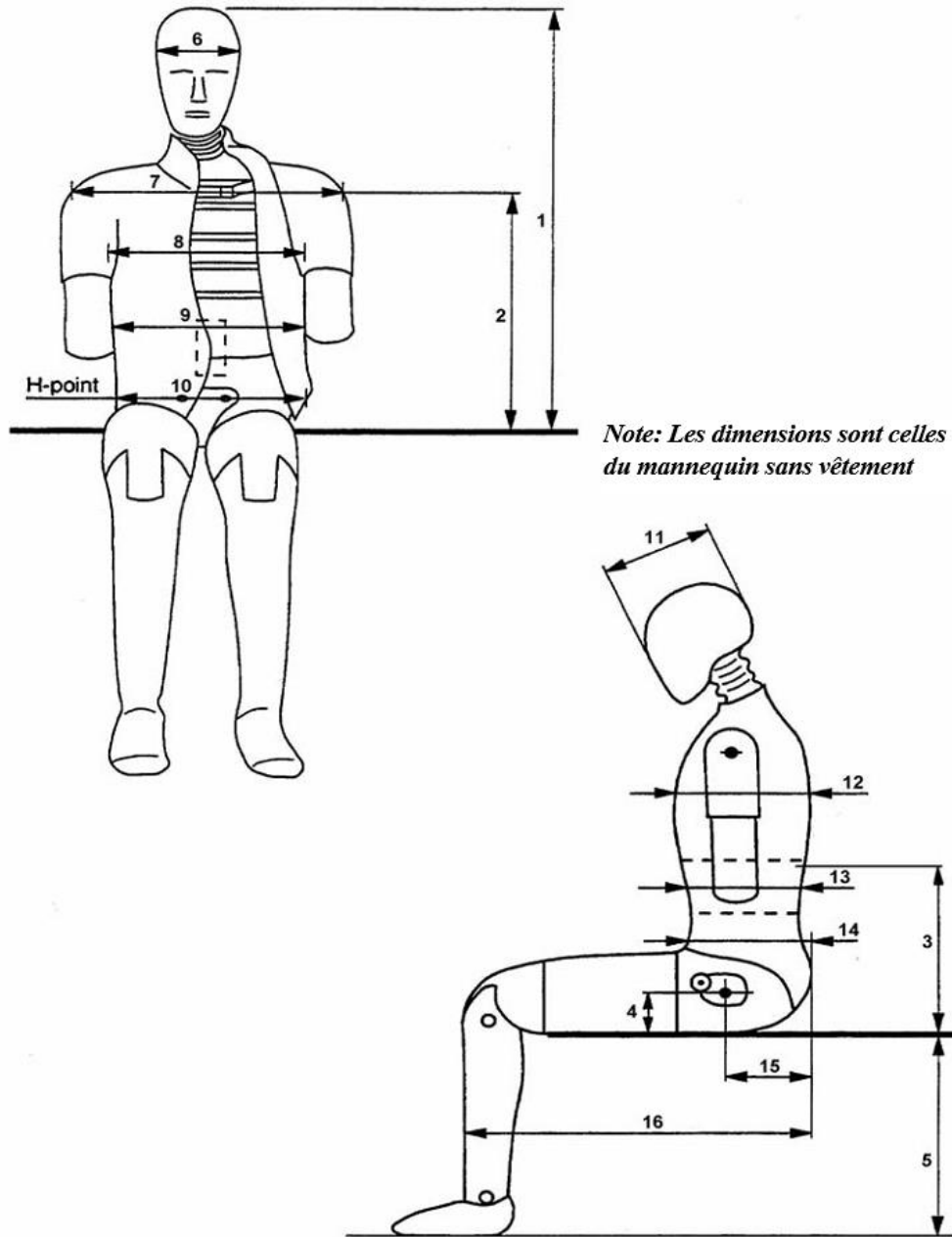
Figure 2 Dimensions principales du mannequin (voir tableau 3)
