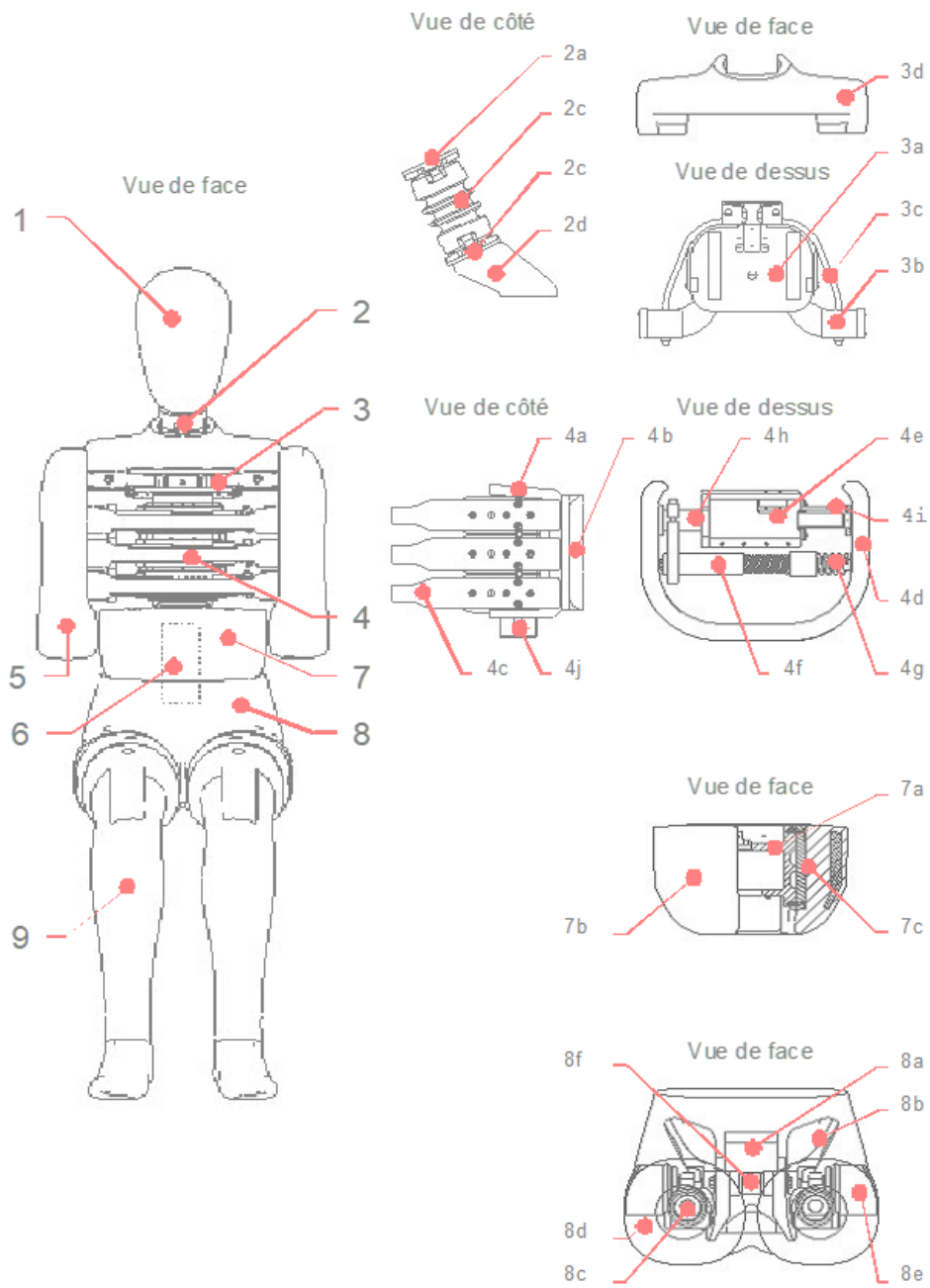
Figure 1 Structure du mannequin pour essais de choc latéral
