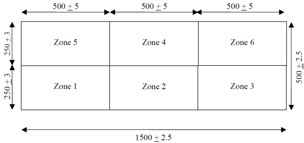
Figure 2 Haut de l'élément de frappe
