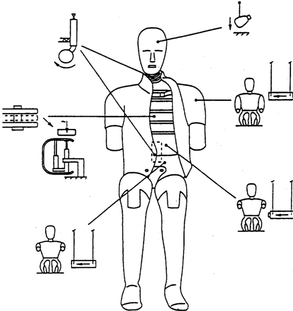
Figure 4 Suspension de l'élément de frappe de 23,4 kg
