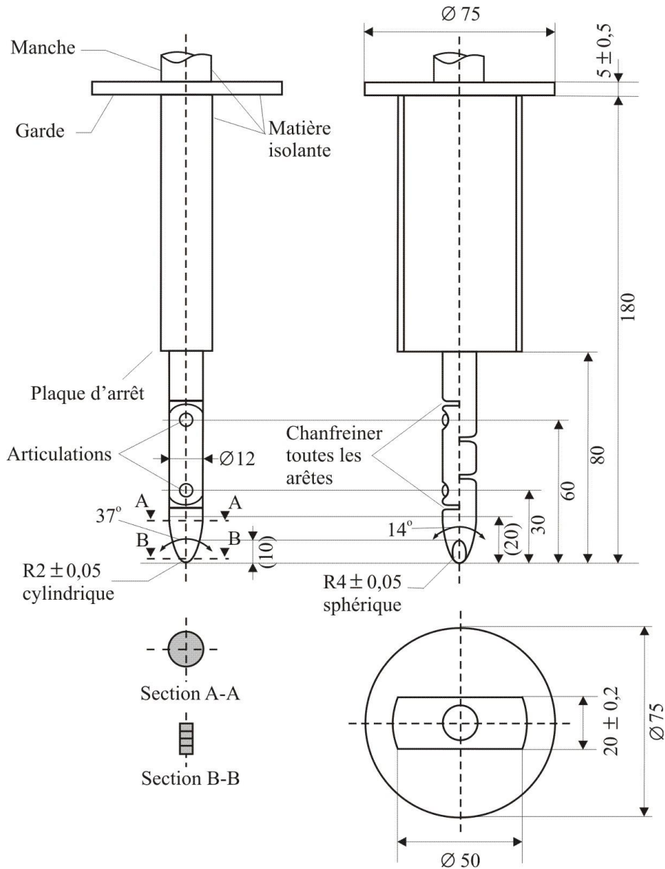
Figure 1 Doigt d'épreuve articulé
