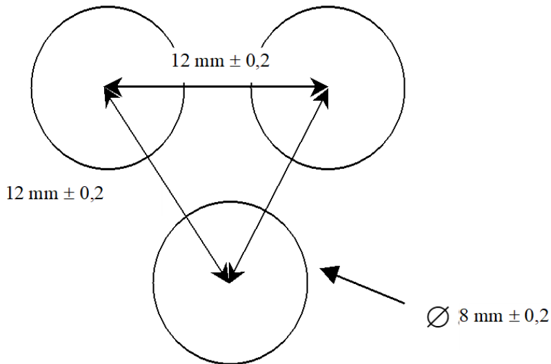
Figure 7 Écartement des orifices de ventilation en quinconce de la plaque arrière
