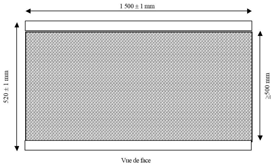
Figure 5 Conception de la plaque arrière
