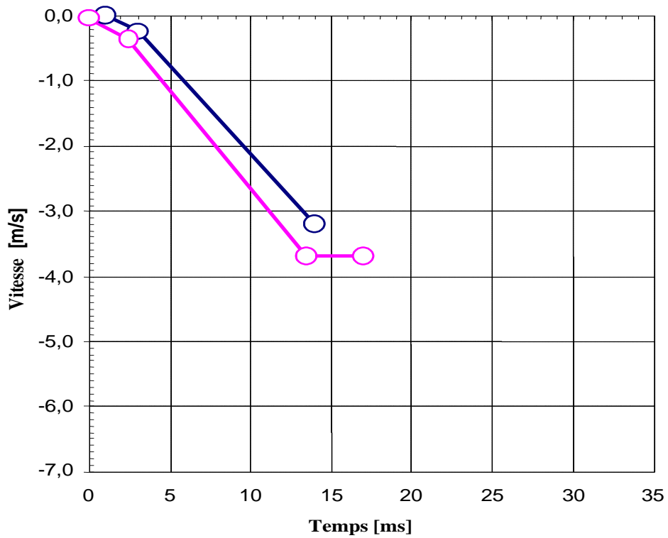
Figure 7 Rapport vitesse/temps du pendule pour l'essai d'homologation du cou
