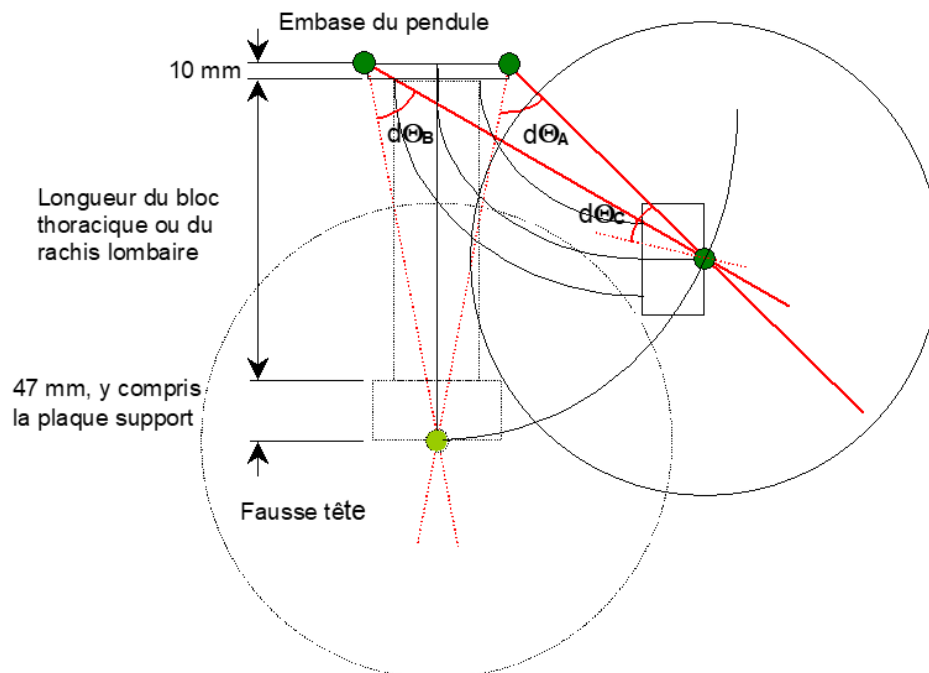
Figure 6 Montage d'essai pour l'homologation du bloc thoracique et du rachis lombaire (angles dθA, dθB et dθC mesurés avec la fausse tête)
