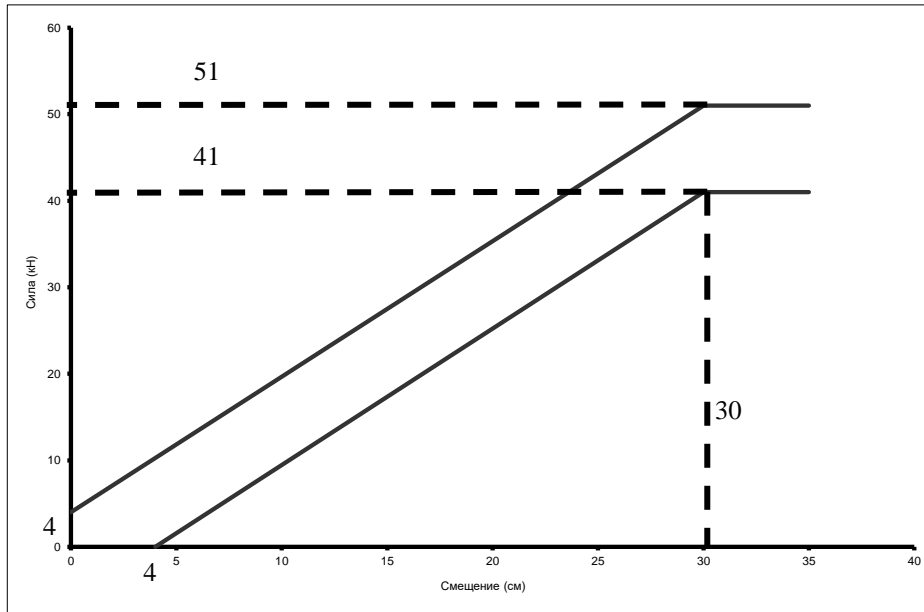
Рис. 1а Блоки 1 и 3
