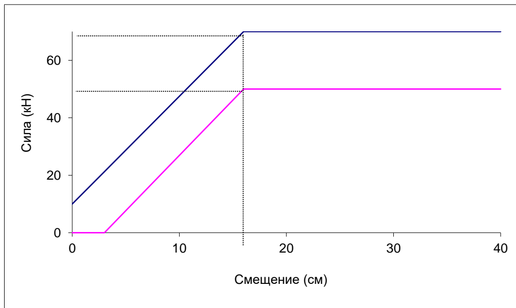
Рис. 2б Блок 2
