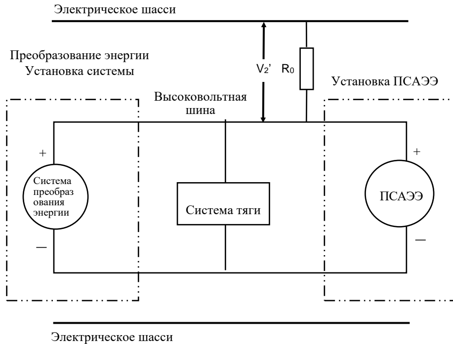
Рис. 4 Измерение V_2'
