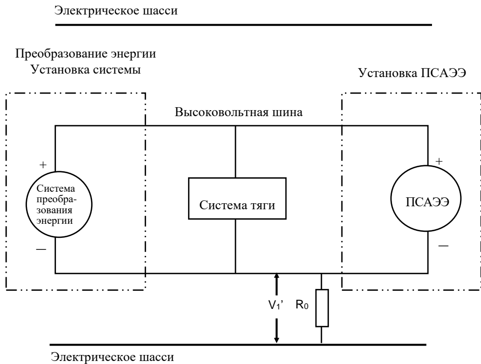
Рис. 3 Измерение V_1'
