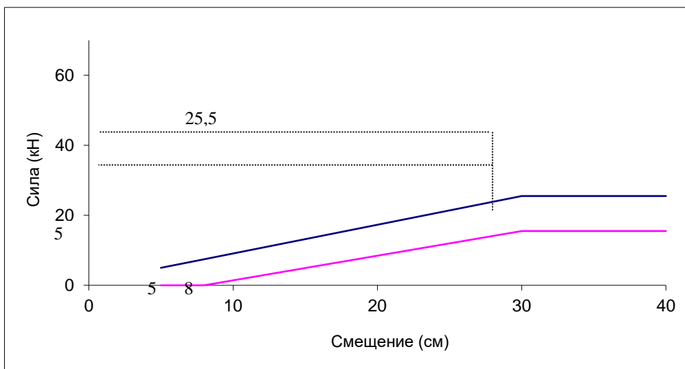
Рис. 2d Блоки 5 и 6
