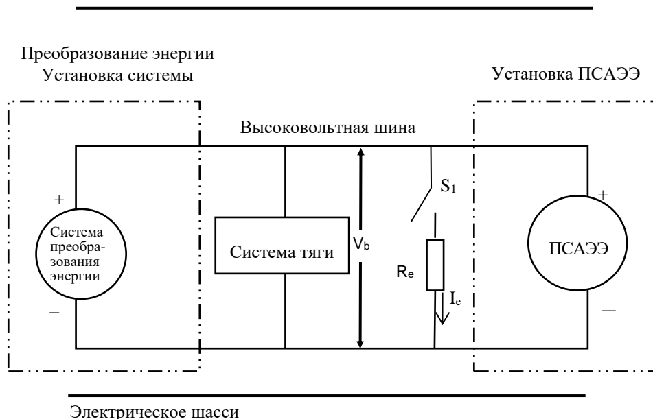
Рис. 2 Примерное измерение количества хранящейся в емкостях X энергии высоковольтной шины
