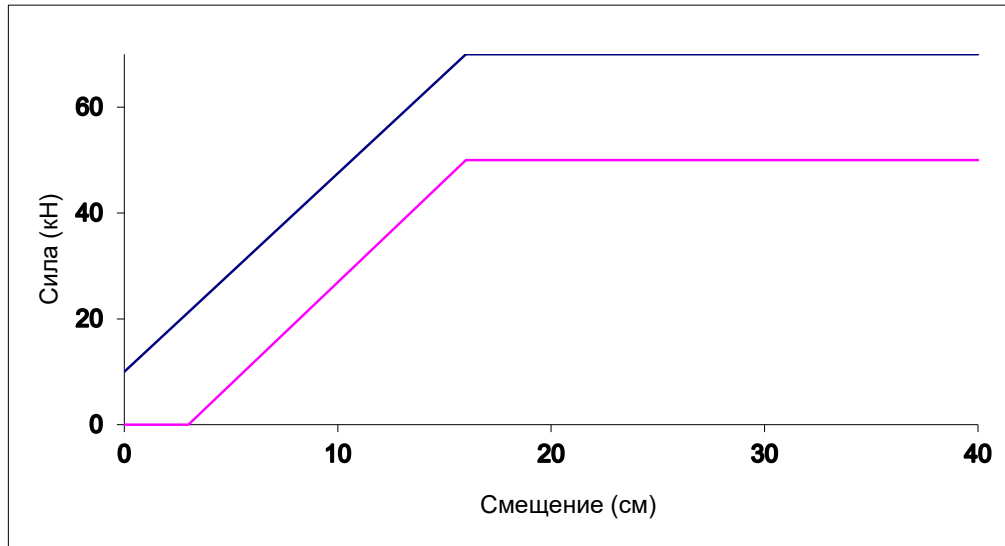
Рис. 2б Блок 2
