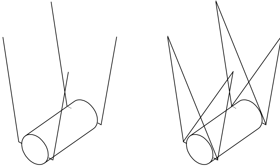
Figure 5 Caractéristiques du pendule cervical conformément au Règlement fédéral n° 49 des États-Unis, chapitre V, partie 572.33
