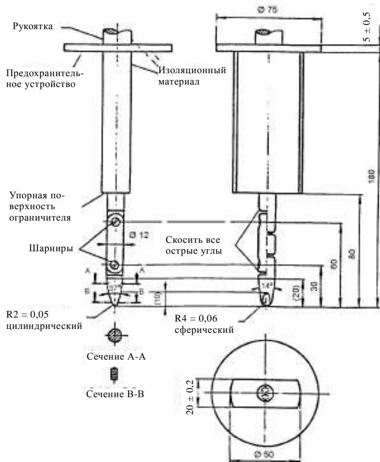
Рис. 12 Шарнирный испытательный штырь
