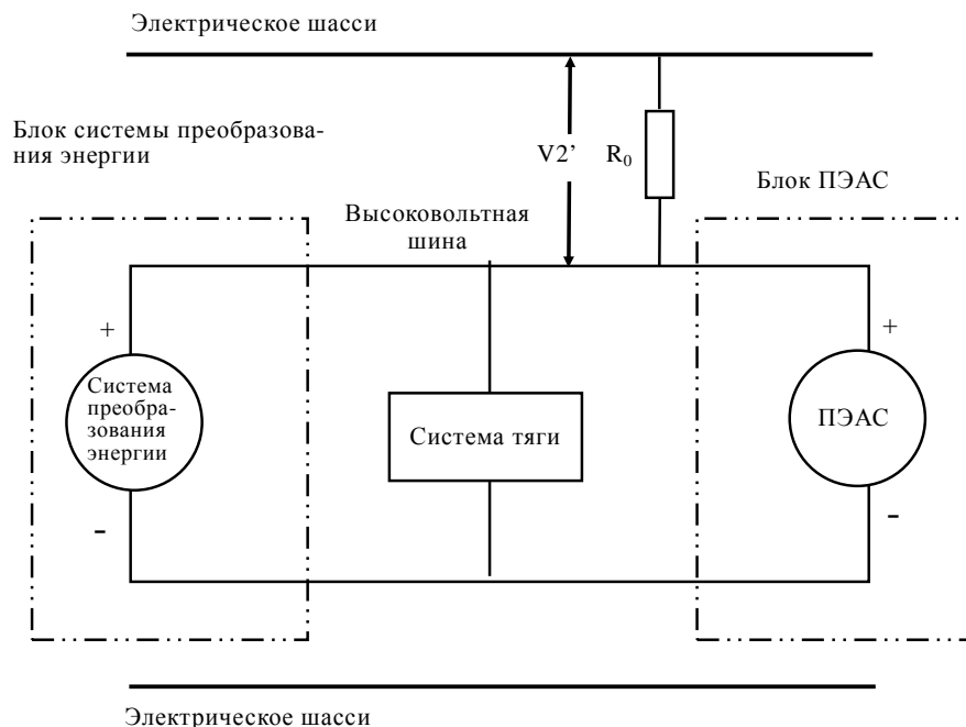
Рис. 11 Измерение значения V_2'
