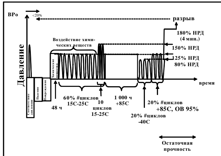
Рис. 2 Проверочные испытания на ресурс прочности (под гидравлическим давлением)
