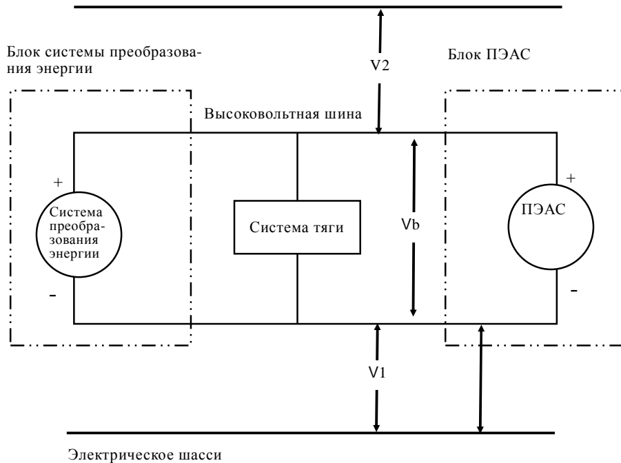
Рис. 14 Измерение значений V_b , V_1 , V_2
