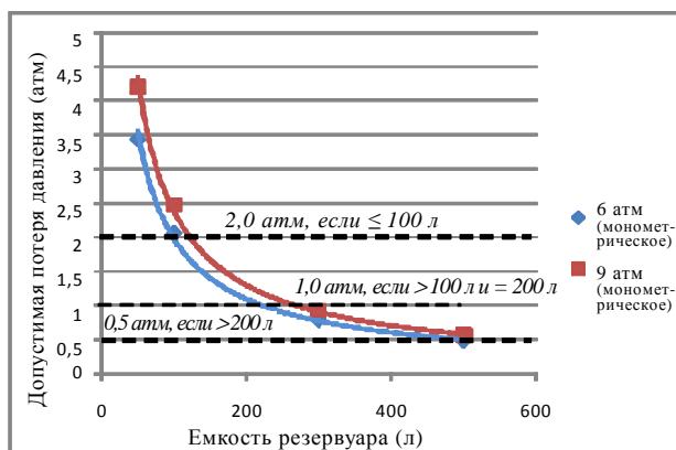
Рис. 5 Допустимая потеря давления в ходе испытания на герметичность СХСЖВ
