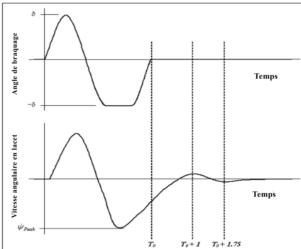
Figure 1 Informations de position du volant et de vitesse angulaire de lacet utilisées pour l'évaluation de la stabilité latérale
