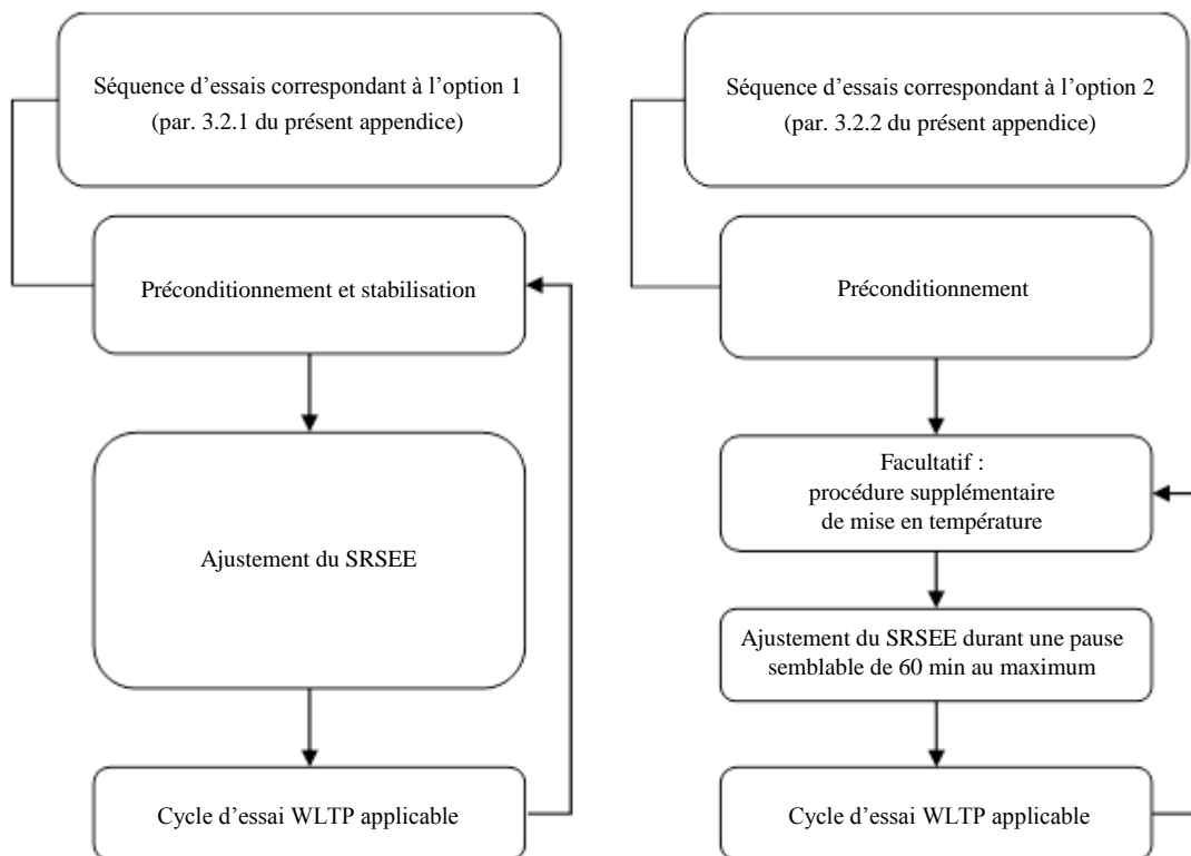
Figure A8.App2/2 Séquences d'essais pour les VHE-NRE et les VHPC-NRE
