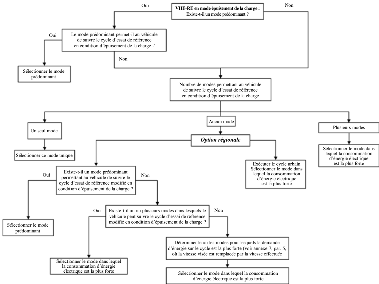
Figure A8.App6/1 Sélection d'un mode de fonctionnement pour un VHE-RE en condition d'épuisement de la charge
