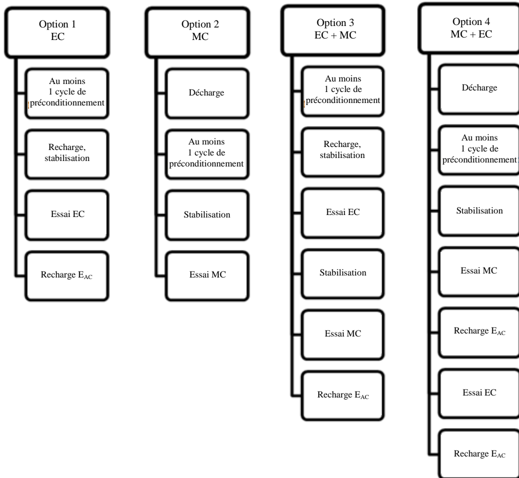
Schéma A8/1 Séquences possibles pour les essais des VHE-RE
