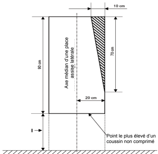
« Figure 7 Intrusion autorisée d'un élément de structure (voir par. 5.7.8.1.3.2) »
